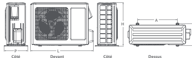
Unité extérieure
